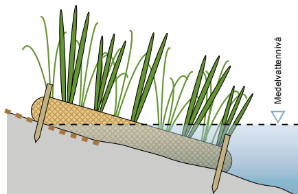
FIGUR 1: Förankring i slänt sker med träspik. Växterna är beroende av kontinuerlig vattentillgång och mattan monteras därför på rätt nivå i förhållande till medelvattennivån.
