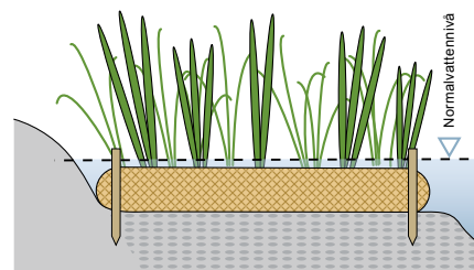
FIGUR 2: I branta slänter kan strandmattan monteras på en hylla som exempelvis byggs upp med grovt makadam.
