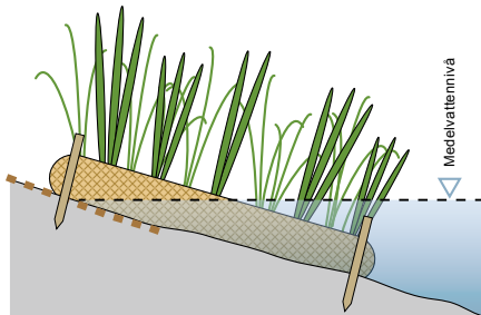
FIGUR 1: Förankring i slänt sker med träspik. Växterna är beroende av kontinuerlig vattentillgång och mattan monteras därför på rätt nivå i förhållande till medelvattennivån.
